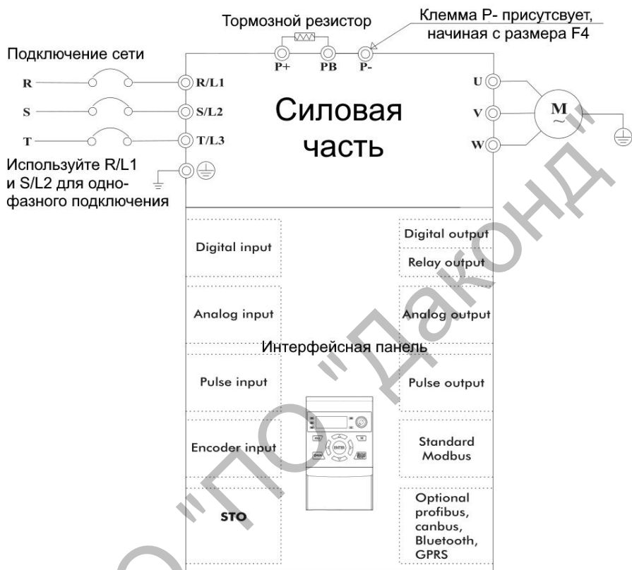
Рис. 3-1 Силовая цепь и интерфейсная панель
