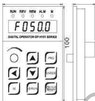
Размеры (мм) 68 (W) x 100 (H) x 25 (D)
