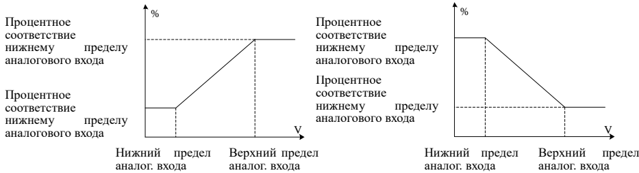
Рис. 6-18 Линейная кривая аналогового входа
