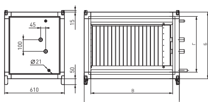
ВЫТЯЖНАЯ часть рекуператора (RGV)
