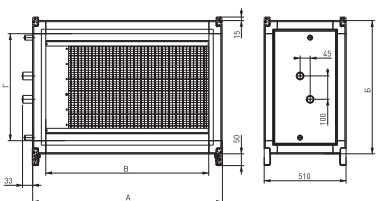
Приточная часть рекуператора (RGP)
